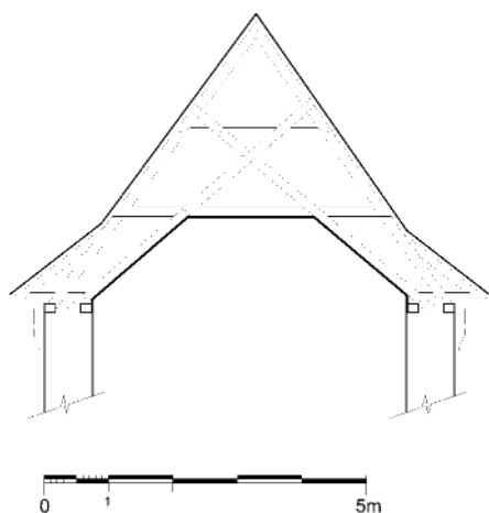
Obr. 14: Praha - Podolí, kostel sv. Michaela archanděla, rekonstrukce možné podoby původního zastřešení a zastropení presbytáře. Sklon a poloha krokvi a poloha hambalků jsou prokazatelné, podoba zastropení a ondřejského kříže je jednou z několika možných variant, podoba paty krovu a jeho uložení na obvodové zdivo je hypotetická (kresba J. Veselý).
