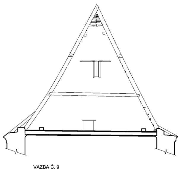
KROV ZÁPADNÍ PŘÍSTAVBY
