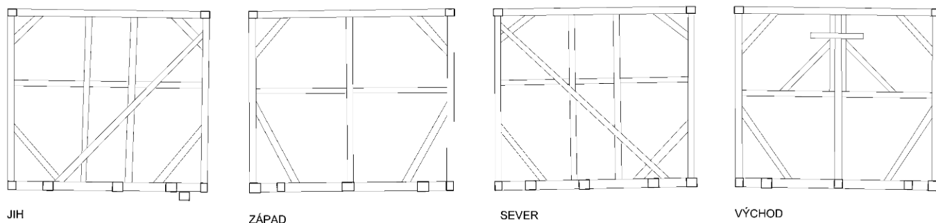
Obr. 18: Praha - Podolí, kostel sv. Michaela archanděla, zaměření zvonice: a – řezy; b – půdorys; c – rámy obvodového pláště (zaměření a kresba J. Veselý).
