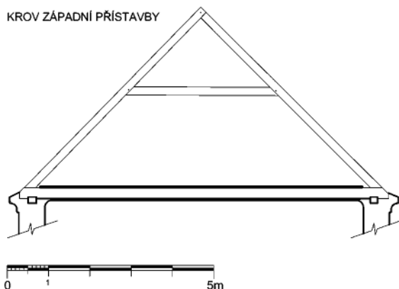
Obr. 7: Praha - Podolí, kostel sv. Michaela archanděla, příčné vazby krovů nad lodí kostela (zaměření J. a P. Veselých, kresba J. Veselý).
